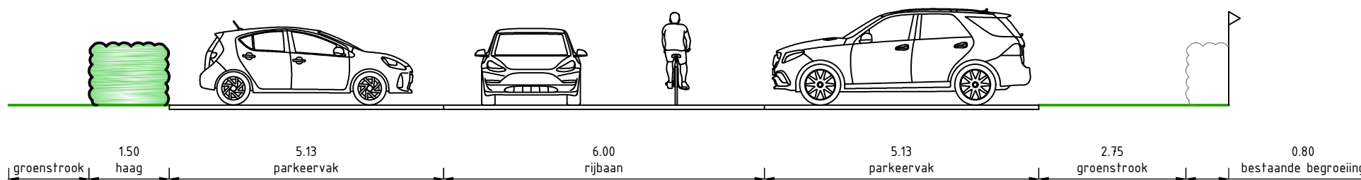
Dwarsprofiel B-B Schaal 1:100
