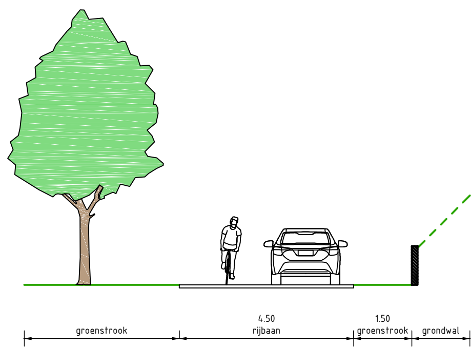
Dwarsprofiel A-A Schaal 1:100
